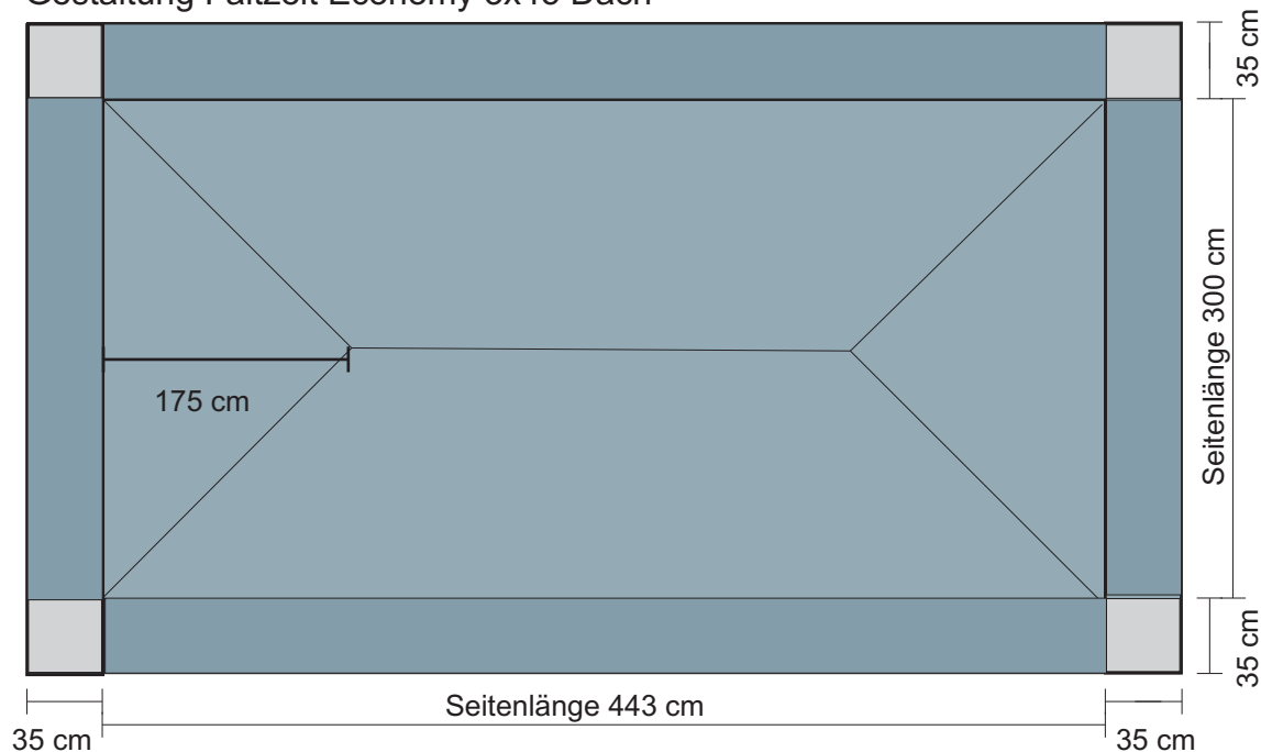
Gestaltung Faltzelt Economy 3x45 Dach
